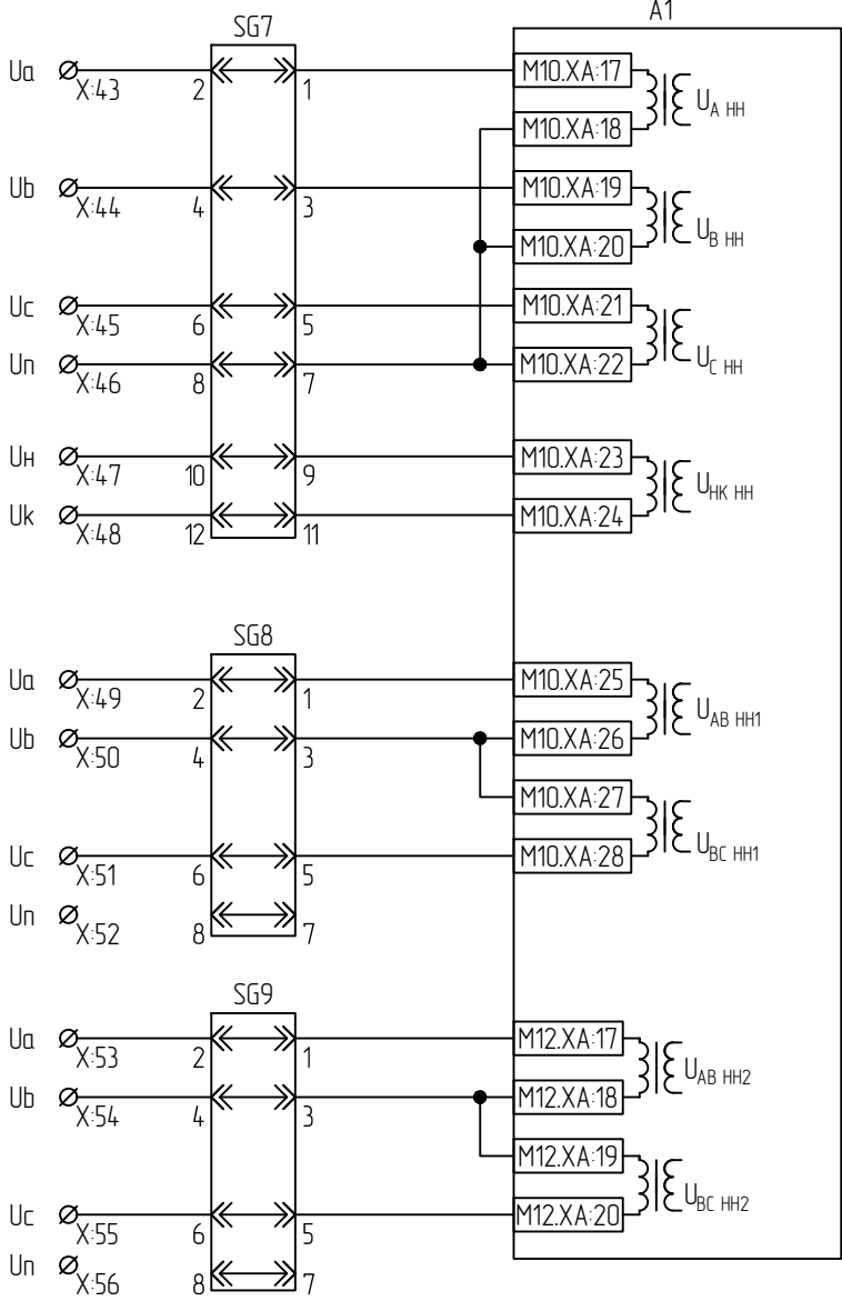
Цепи переменного и напряжения A1
